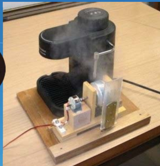
簡易型蒸気発電機(加島篤氏製作)
